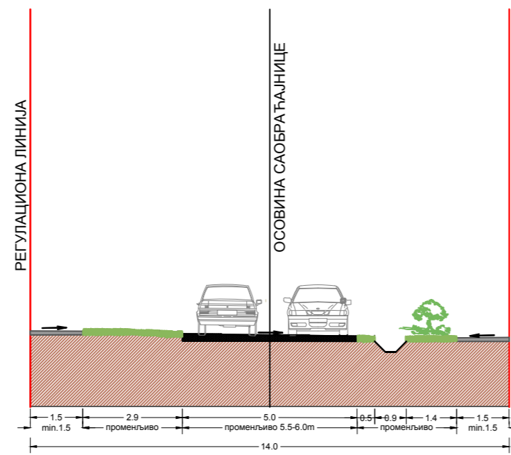
Пресек 6-6
