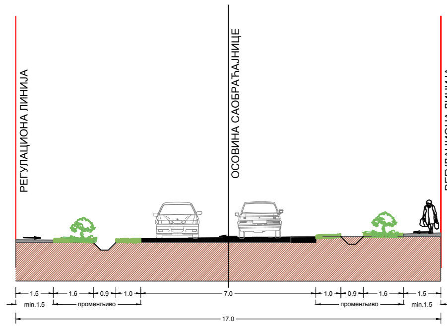
Пресек 1-1
