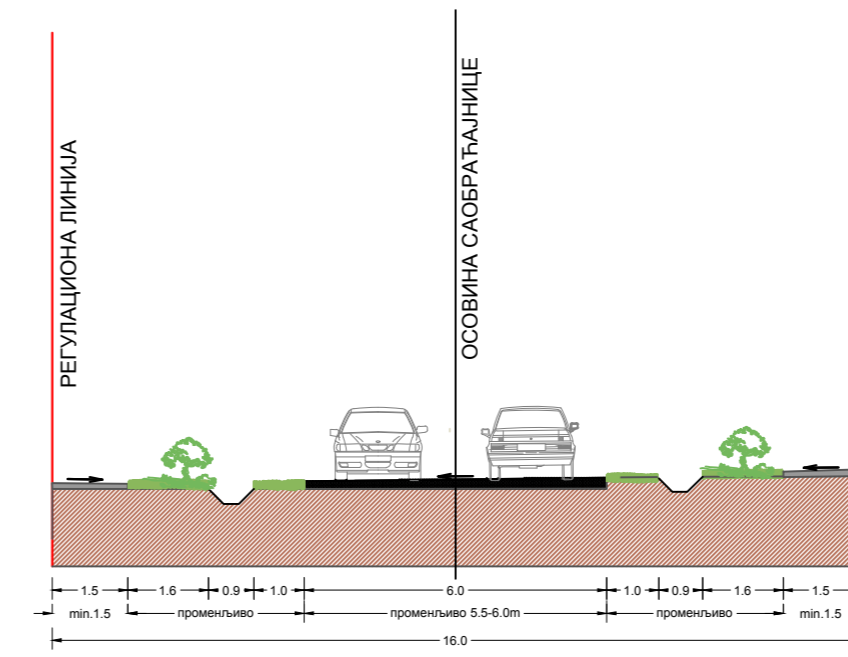
Пресек 3-3
