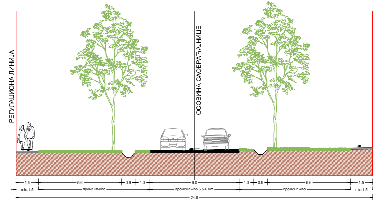
Пресек 2-2
