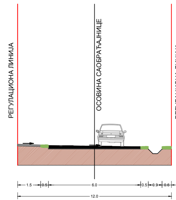
Пресек 4-4
