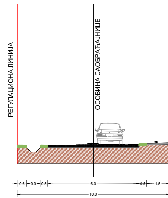
Пресек 5-5
